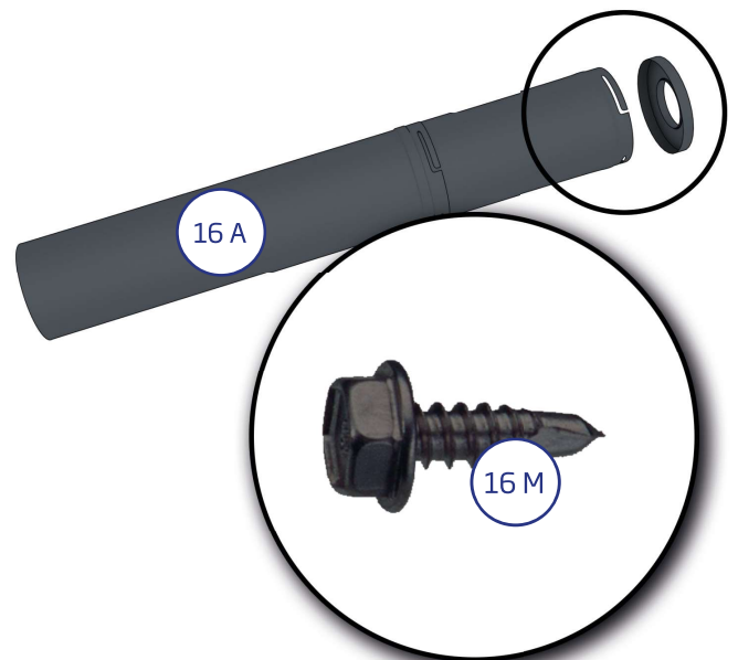
10. Kiinnitä yläpäätty teräspiippuun ( 16 A ) kolmella itseporautuvalla ruuvilla ( 16 M ). Ruuvit porataanpellin läpi.
