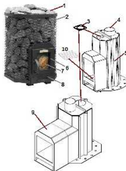
Рисунок 1. Части печи
