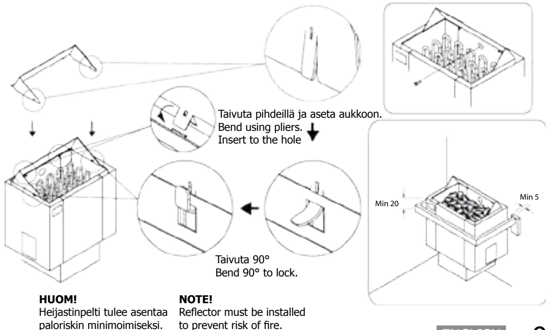
Kuva 2 | Löylynohjaimen asentaminen Fig. 2 | How to install Reflector
