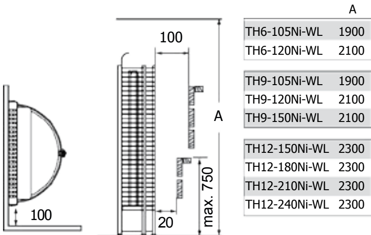
Kuva 2 | Minimisuojaetäisyydet (mm) Fig. 2 | Minimum safety distances (mm)
