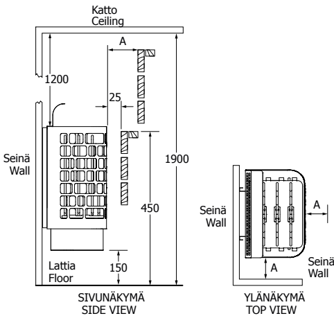
Kuva 1 | Minimisuojaetäisyydet (mm) Fig. 1 | Minimum safety distances (mm)
